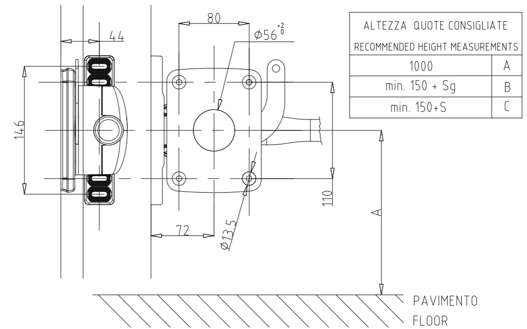
SCHEMA FORATURE PER KIT PORTA 3 PUNTI DRILLING DIAGRAM FOR 3 POINT DOOR KIT
