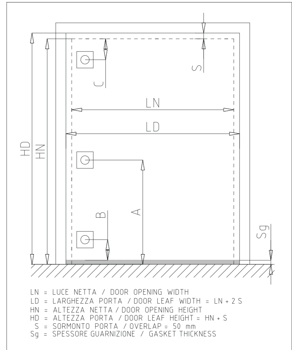
SCHEMA FORATURE PER KIT PORTA 3 PUNTI DRILLING DIAGRAM FOR 3 POINT DOOR KIT
